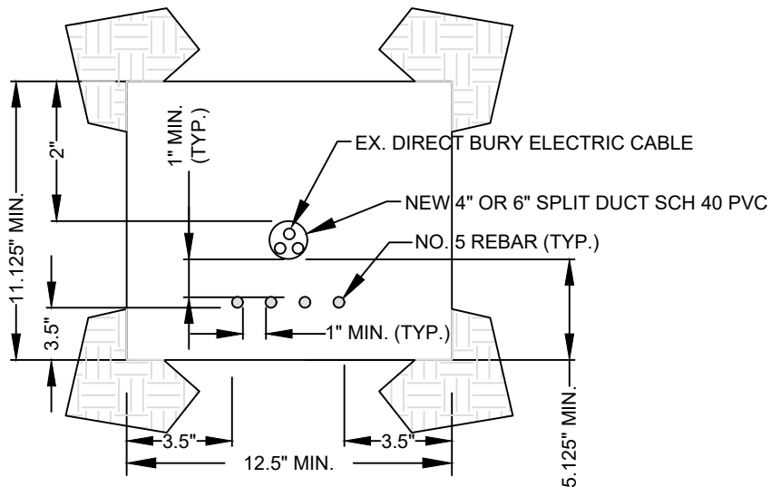
DETAIL 1 N.T.S.
