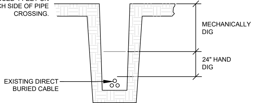
UNCOVERING EXISTING CABLE N.T.S.
