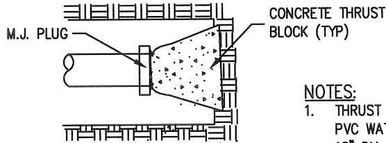
DEAD END
